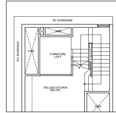
LOFT - PLAN
